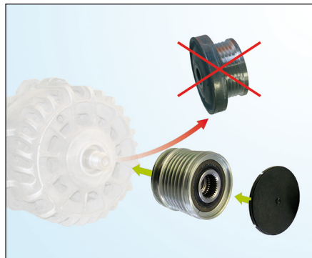
Imagen 3: Sustitución
