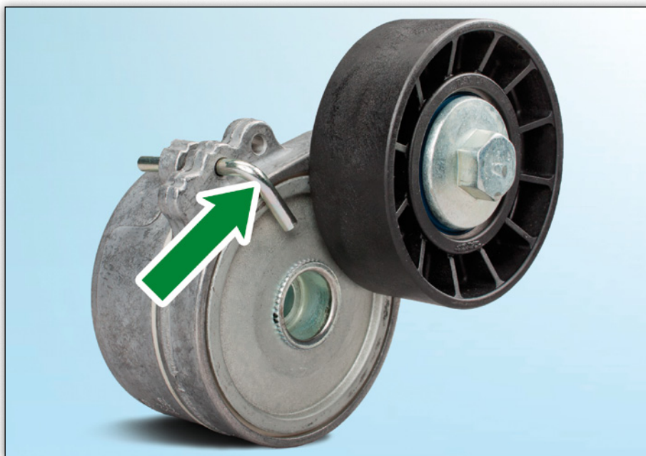
Fig. 1: Brazo tensor INA 534 0110 20 con pasador de seguridad
