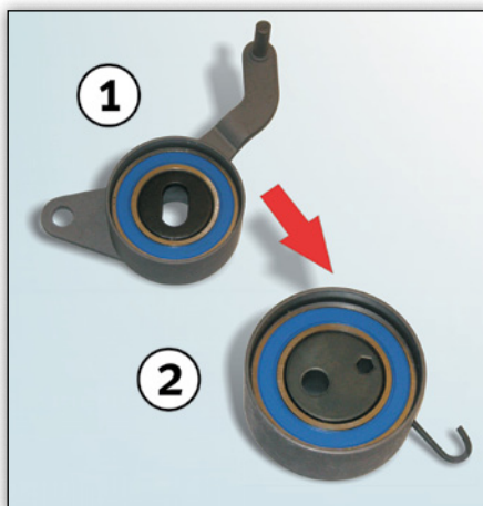
Fig. 1: Polea tensora sustituida 531 0166 20 (1) y sucesora 531 0819 10 (2)
